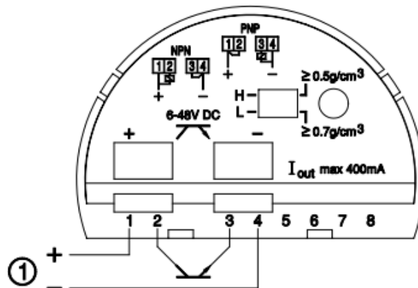
图8 晶体管(NPN/PNP)输出方式
