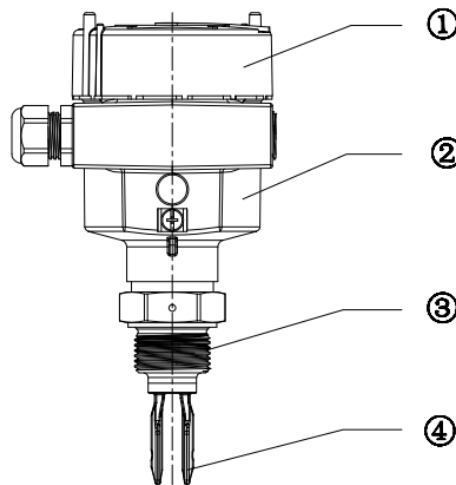
图 1 Ring-11 整体结构图
