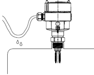
图 4 防潮安装
