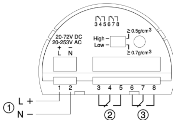
图 5 继电器输出方式
