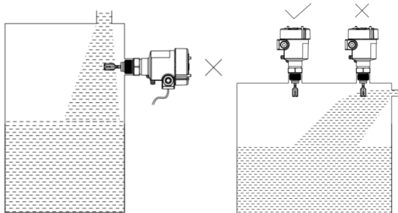
图 3 避开入料口的安装示意图
