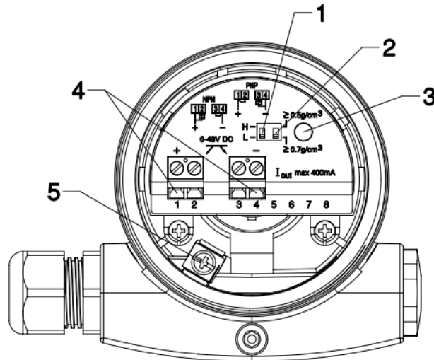
图 14 晶体管(NPN/PMP)输出方式
