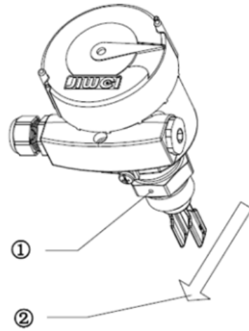
图 2(b) 介质流动方向
