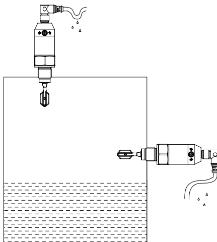
图4 防潮安装
