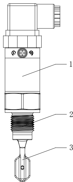
图 1 Ring-21 整体结构图
