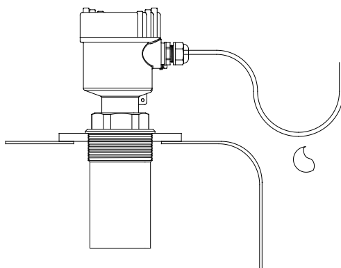
图 6 防潮安装
