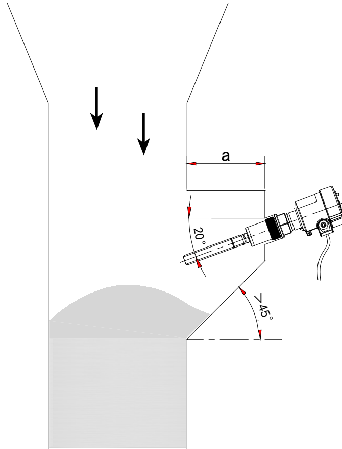
图 3 壁龛式安装示意图
