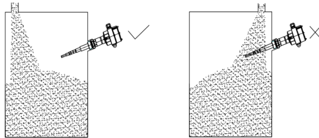
图5 避免入料口的安装示意图
