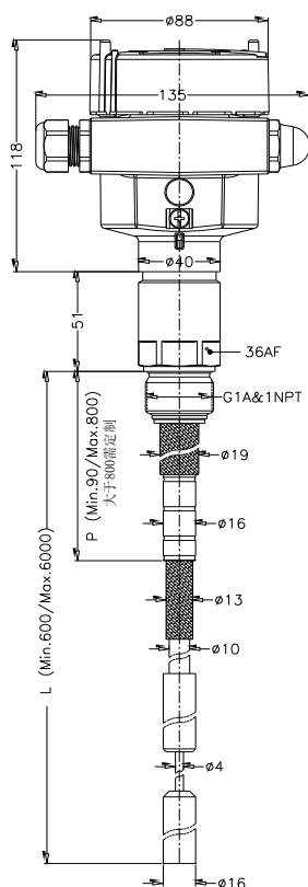
Cape-11R 缆绳型
