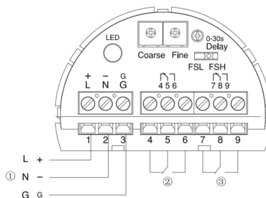
图8 接线示意图
