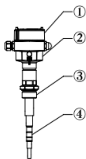
图 1 Cape-11 整体结构图
