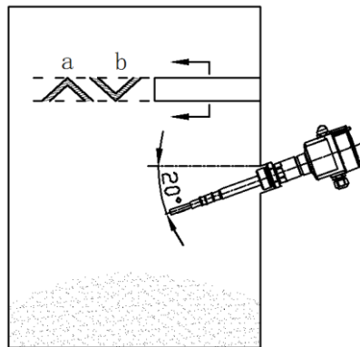
图 2 挡板式安装示意图
