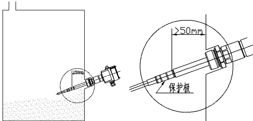
图7 保护极插入深度
