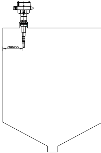
图 4 垂直安装示意图
