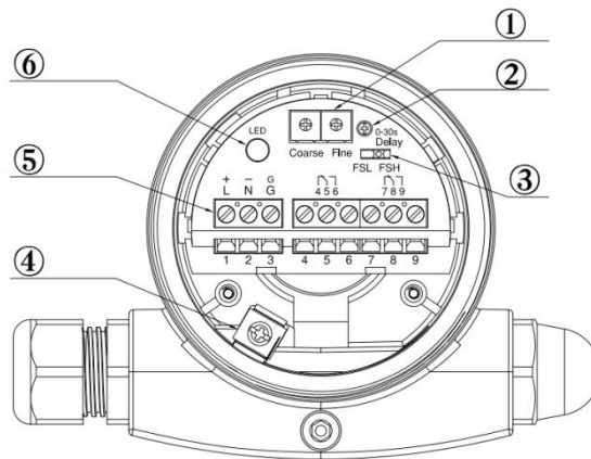
图 9 内部结构图
