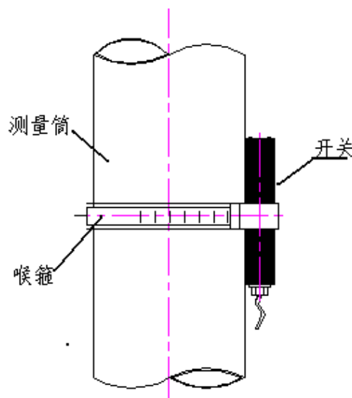
图 1 SW-11 磁开关安装示意图
