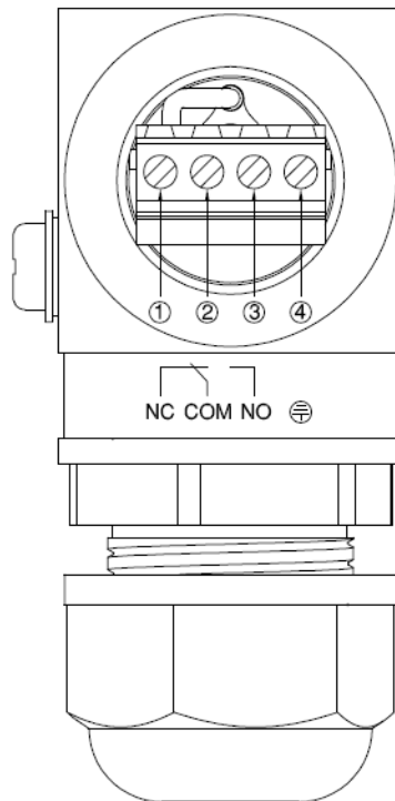
图 5 SW-21 接线图
