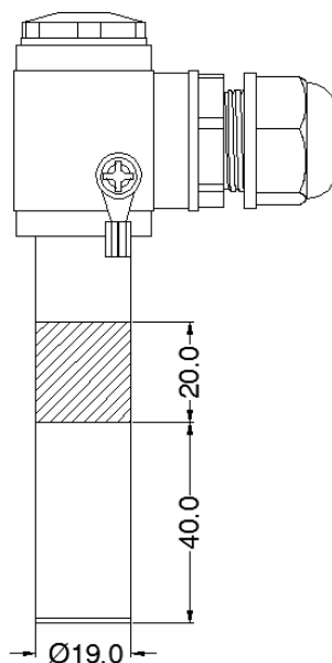
图 4 SW-21 动作点范围
