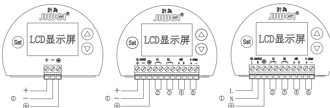
图 7 接线图
