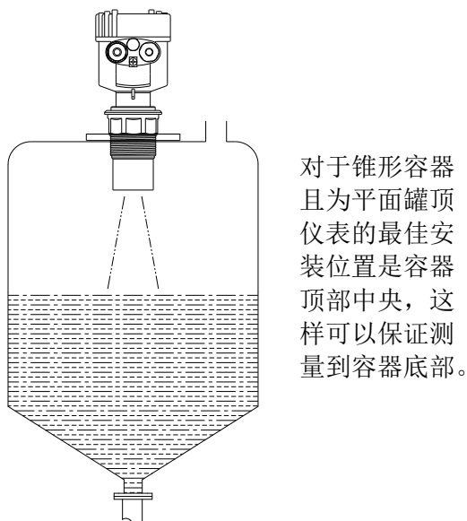
图 5 锥形罐安装示意图
