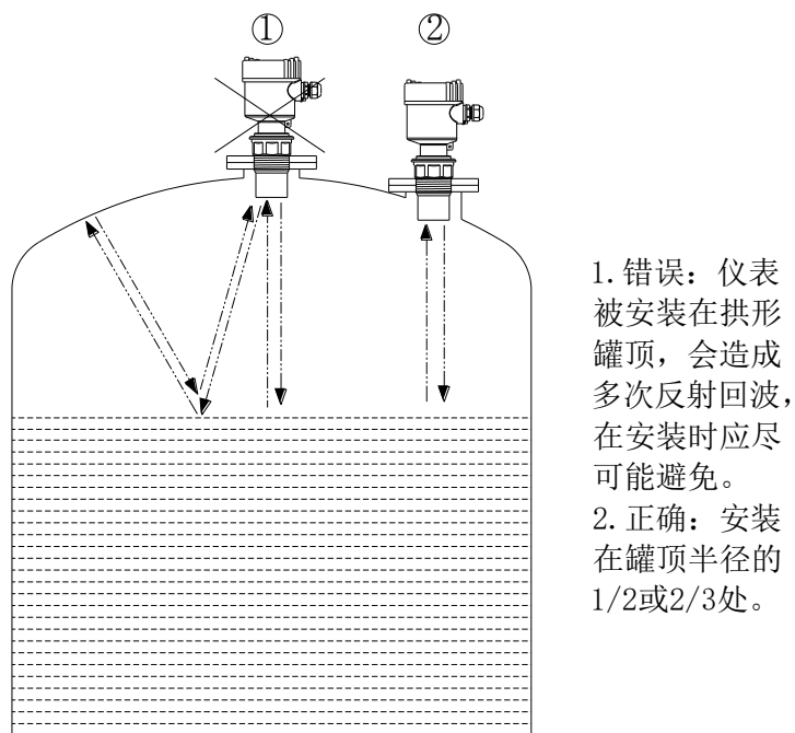
图 4 拱形罐安装示意图
