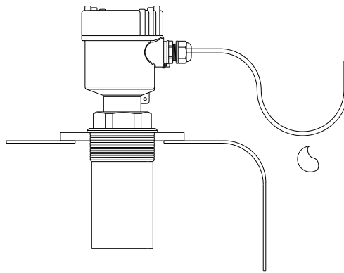
图 6 防潮安装
