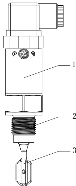
图 1 Ring-21 整体结构图
