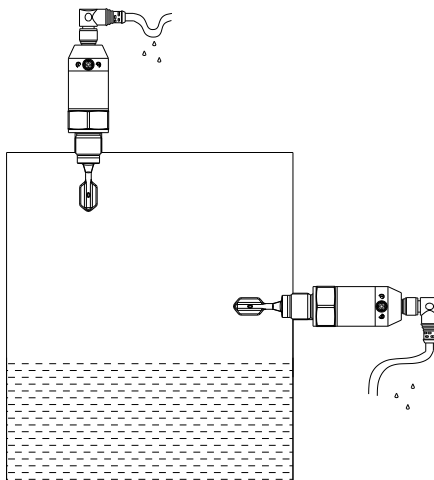
图 4 防潮安装
