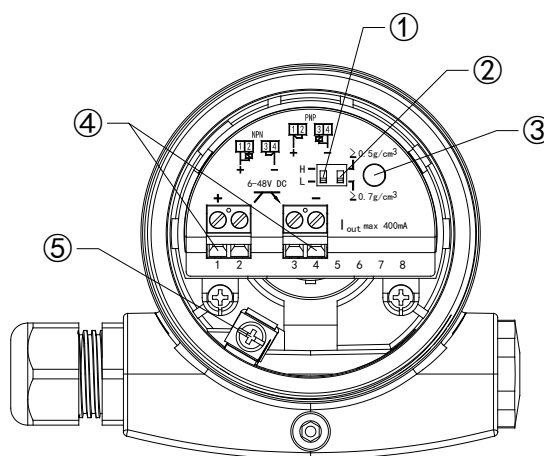
图 14 晶体管(NPN/PMP)输出方式
