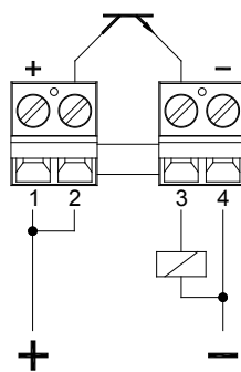
图 10 PNP 工作方式
